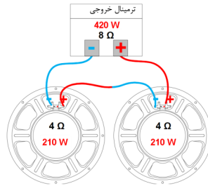
اتصال سری دو بلندگوی ۲۱۰ وات
